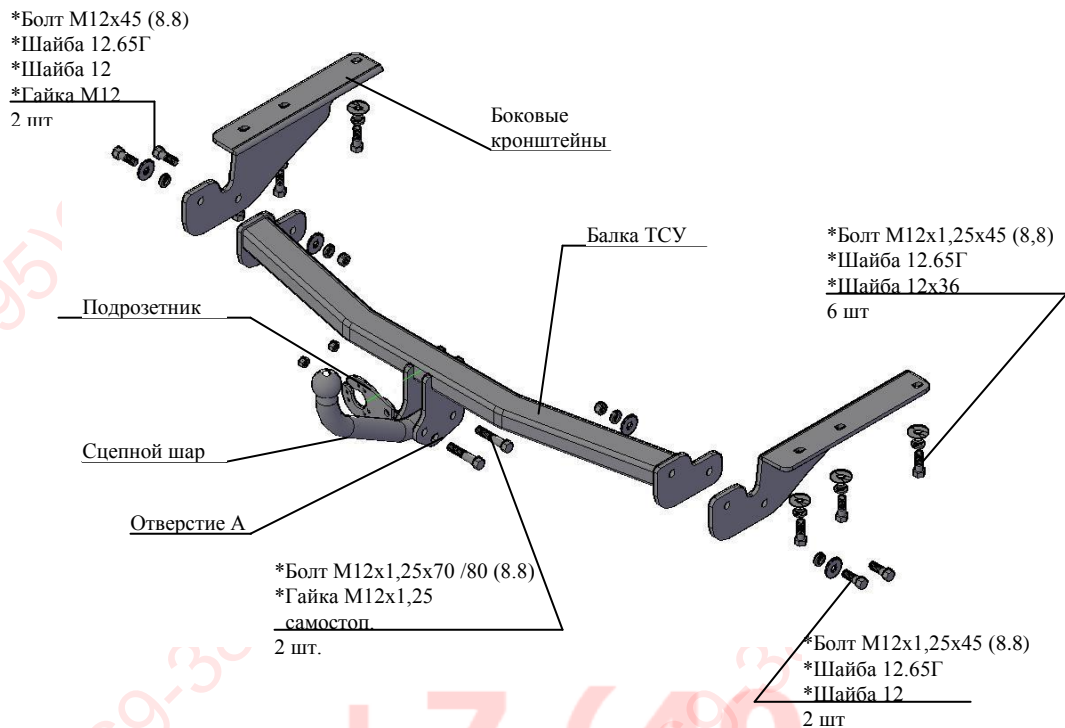
Рис.1 Тягово-сцепное устройство 7830.
